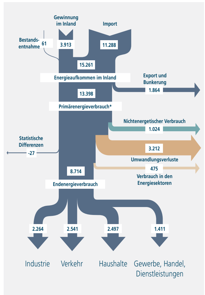
Energieflussbild für die Bundesrepublik Deutschland (2009, in Petajoule, 30 P ca 1 Mio t SKE)
